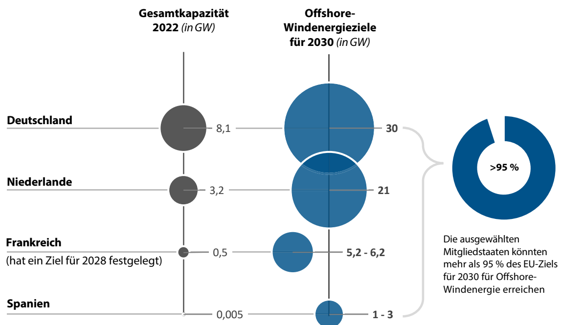
Abbildung 4 – Überblick über die nationalen erneuerbaren Offshore-Energien im Jahr 2022 und Ziele für 2030 (in GW)
