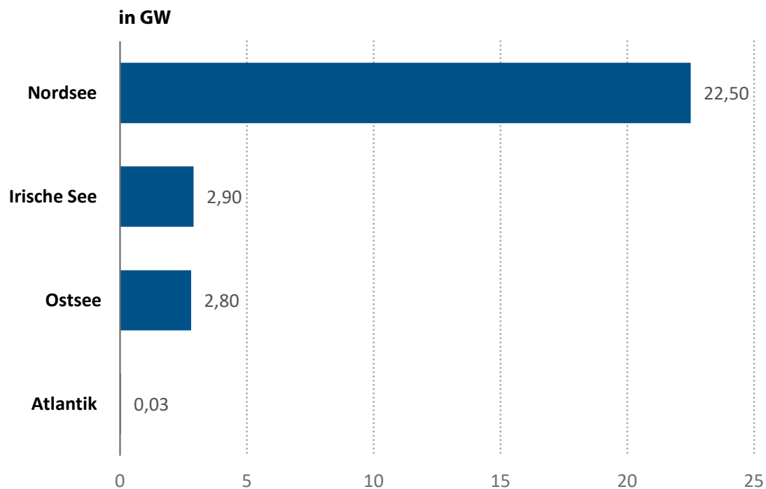
Abbildung 5 – Offshore-Windenergie nach Meeresbecken in Europa (EU- und Nicht-EU-Länder) Ende 2021
