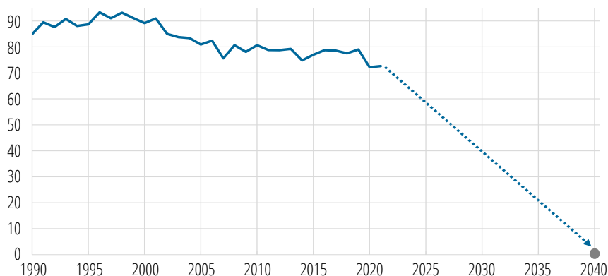
CO 2 -Emissionen Bayern gesamt in Mrd. Tonnen pro Jahr
